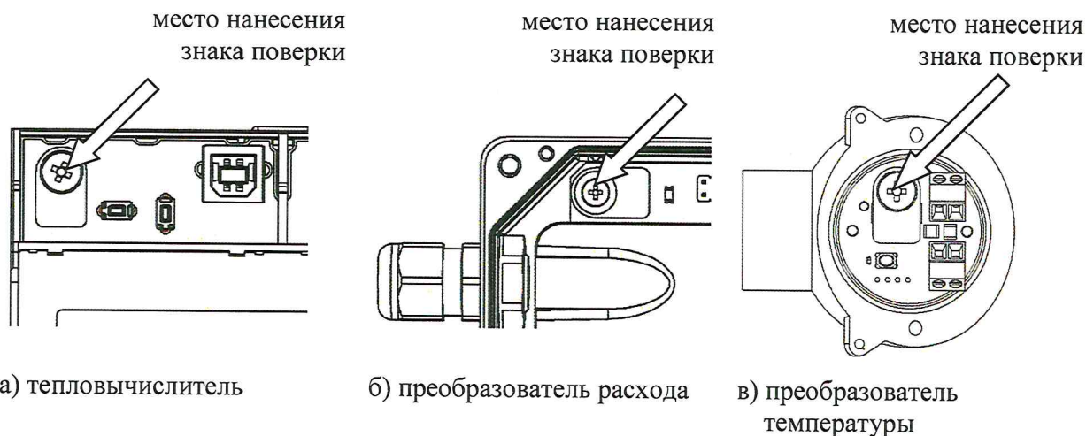
Рисунок 2 – Схема пломбировки от несанкционированного доступа, обозначение мест нанесения знака поверки
