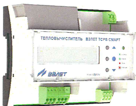
а) вид тепловычислителя «ВЗЛЕТ ТСРВ СМАРТ»
